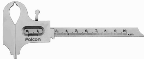
گیج اندازه گیری با قفل اهرمی | F 100.010
